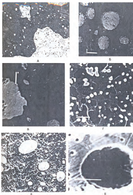
Рис 2.Микроструктура отожжённых при 873К сплавов системы Pd - Er - Fe
