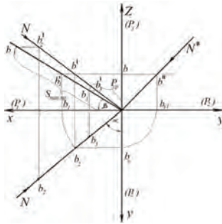
Рисунок 1 – комплексный чертеж условной точки V_1 , адекватной параметрам проекта P_1=40б, P_2=P_3=30б (дифференцированная модель)
