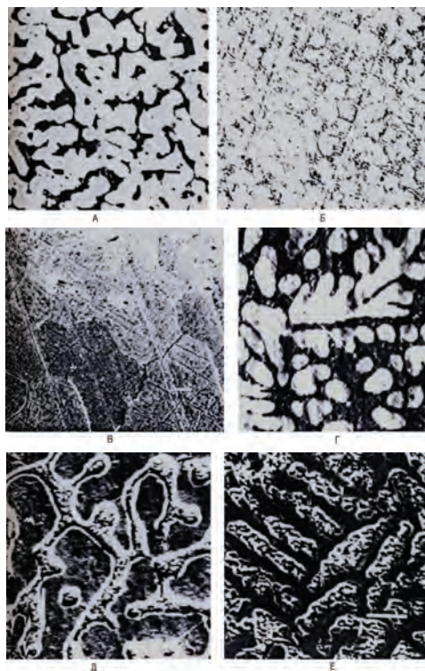
Рис 3. Микроструктура отожжённых при 873К сплавов системы Pd - Er – Fe
