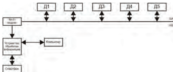
Рисунок 1 – Структурная схема
