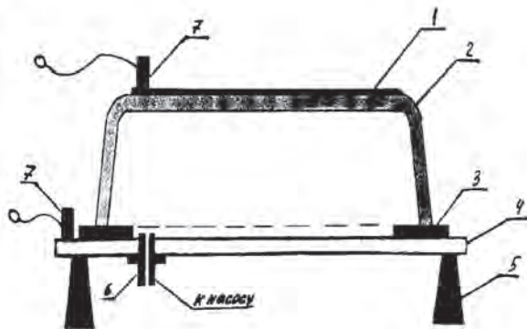
Рис.2 (Устройство газоразрядной камеры. 1) Верхний электрод. 2) Корпус камеры. 3) Герметизирующая прокладка 4) Основание (нижний электрод) 5) Подставка 6) Трубка для соединения со шлангом вакуумного насоса 7) клеммы для крепления проводов).
