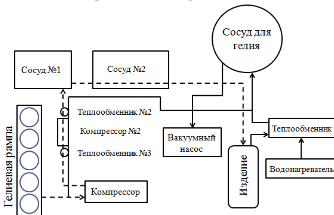
Рисунок 1 – Схема предлагаемой установки
