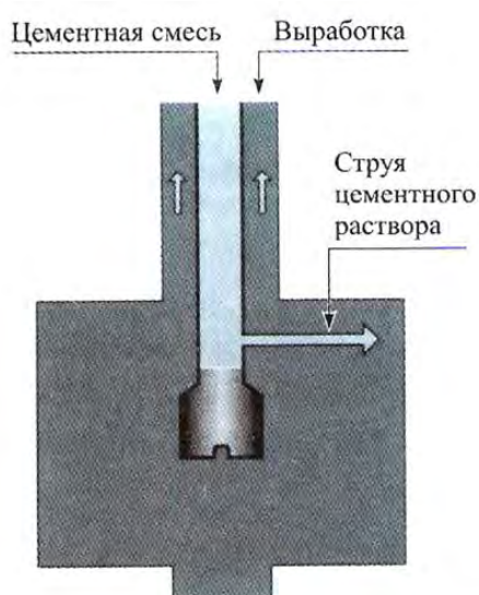
Рис. 2. Схема однокомпонентной струйной технологии цементации методом струйной технологии
