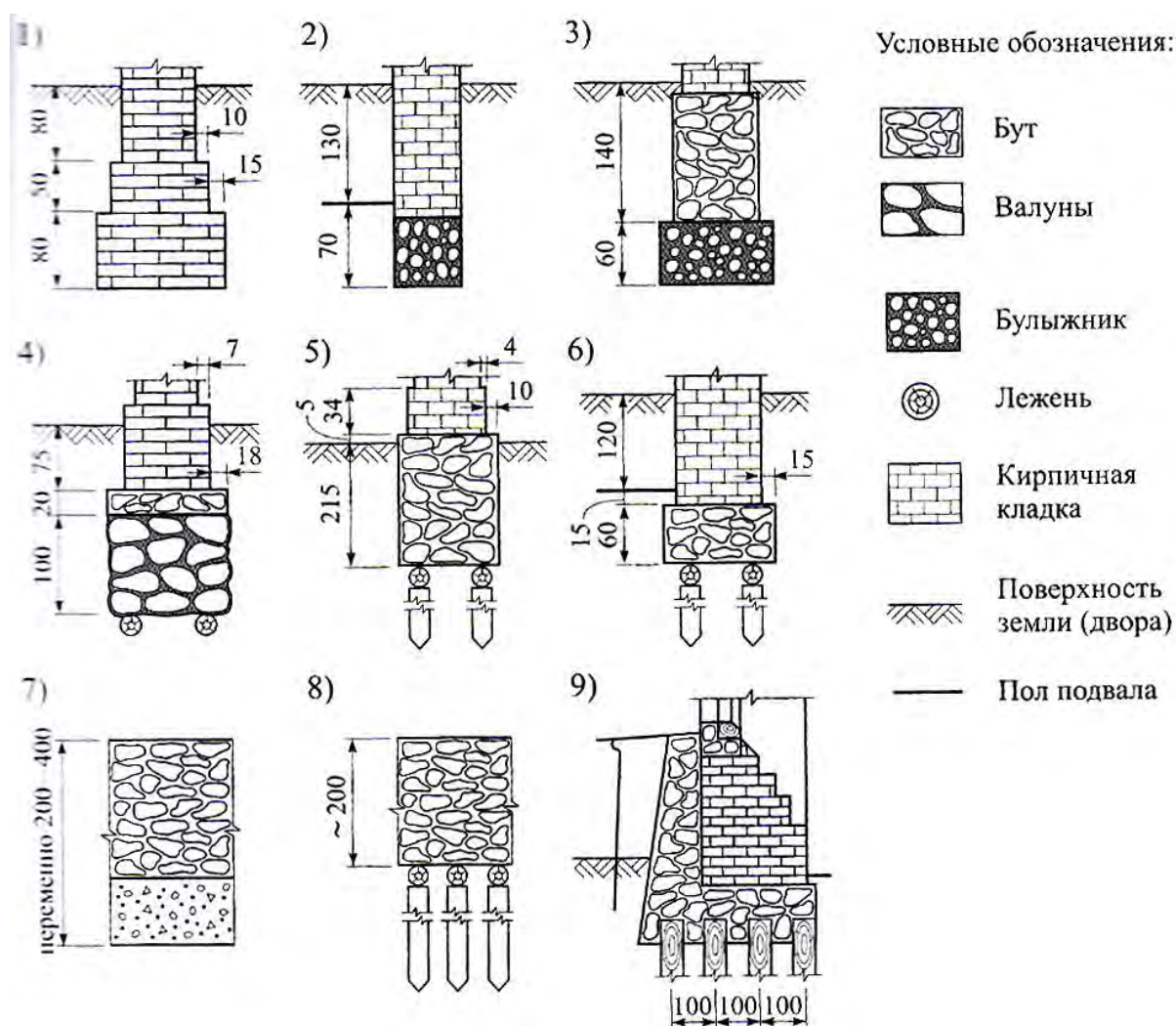
Рис.1. Примеры некоторых типов фундаментов старинных зданий Санкт-Петербурга по результатам обследований (по С.Н. Сотникову[5,6])
