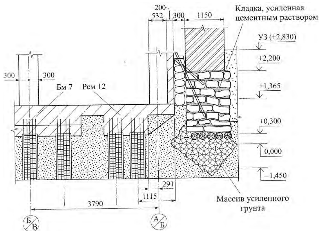
Рис. 4. Узел примыкания балки к фундаменту, закрепленному по методу jet grouting
