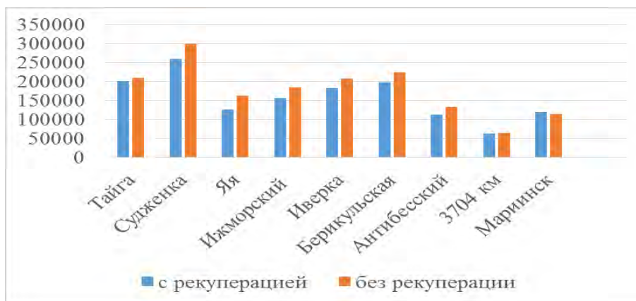
Рисунок 1 – Расход электрической энергии на тягу поездов по счетчикам
