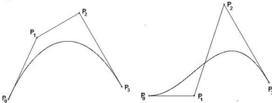
Рисунок 2 – Влияние положения опорных вершин на форму кривой Безье
