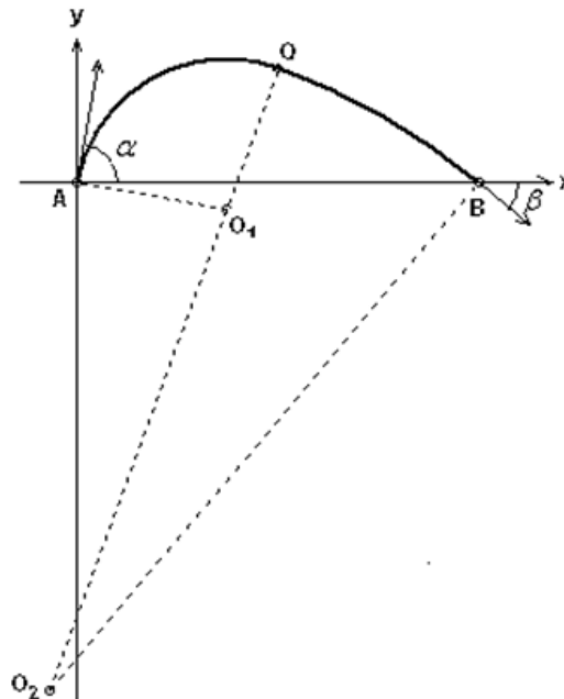
Рисунок 1 – Построение сопряженных дуг с минимальным скачком кривизны. Углы наклона касательных \alpha = 80^\circ , \beta = 40^\circ .
