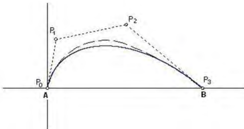
Рисунок 3 – Аппроксимация сопряженных круговых дуг кубической кривой Безье.
