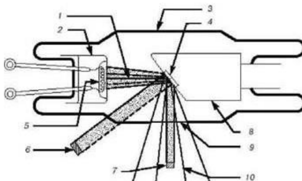
Рисунок 1 – Трубка Кулиджа
