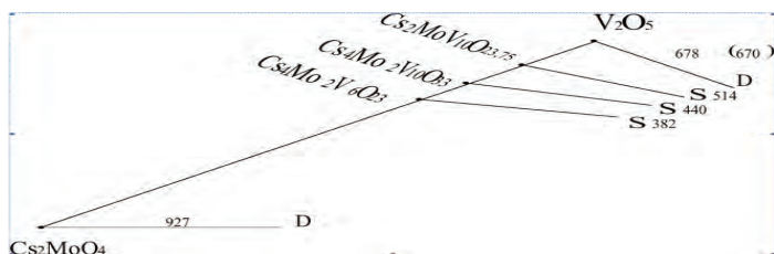
Рис. 2. Схема фазовой диаграммы системы \text{Cs}_2\text{MoO}_4 - \text{V}_2\text{O}_5
