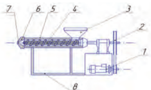
Рисунок 1 - Общий вид и схема лабораторного пресс - экструдера ХР - 3
