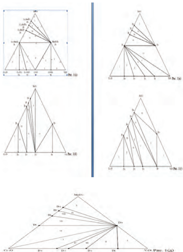
Рис. 1. Топологический образ фазовой диаграммы системы Cs_2O - V_2O_5 - MoO_3 и ее предварительная триангуляция
