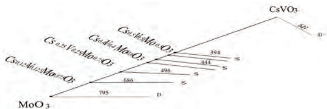
Рис. 1. Схема фазовой системы \text{MoO}_3 - \text{CsVO}_3
