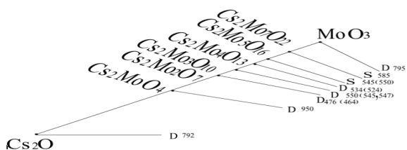
Рис. 2. Схема фазовой диаграммы системы Cs_2O - MoO_3
