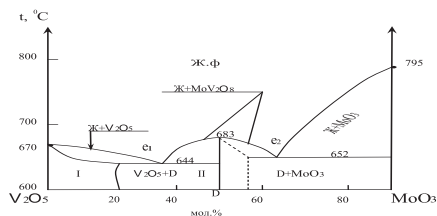
Рис. 3. Фазовая диаграмма системы V_2O_5 - MoO_3 : (I – Mo_{5x}V_{10-6x}O_{40} ; II – MoV_2O_8 )
