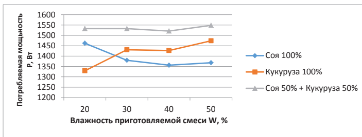
Рисунок 4 - Зависимости потребляемой мощности от исходной влажности продукта
