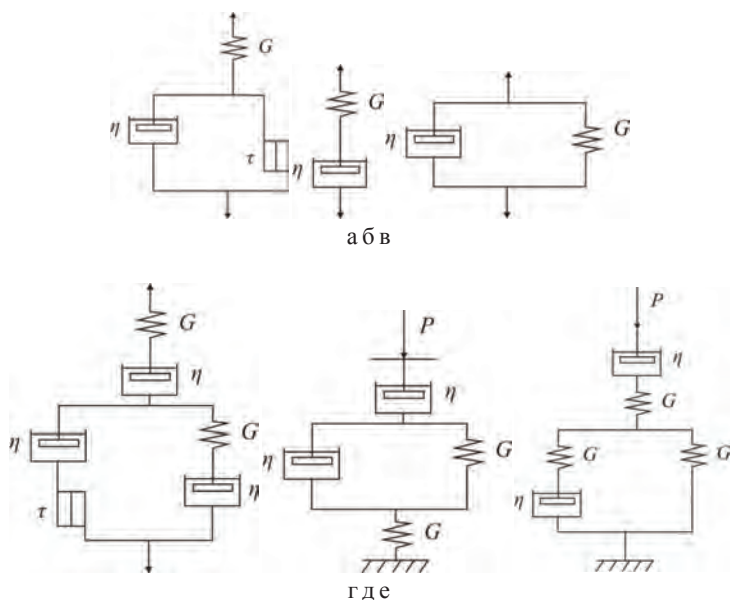
а – Модель упруго - вязкопластического тела Бингама; б – Модель Максвелла; в – модель Кельвина - Фойгта; г – модель Широ́ва; д – модель Особова; е – модель Долгова
