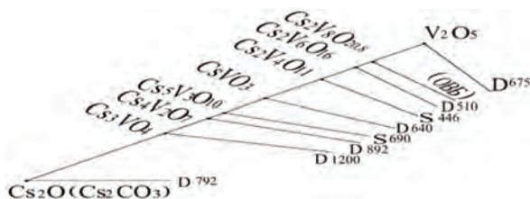
Рис. 1. Схема фазовой диаграммы системы \text{Cs}_2\text{O}(\text{Cs}_2\text{CO}_3) - \text{V}_2\text{O}_5 . ОВБ – оксидная ванадиевая бронза
