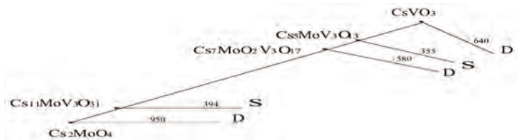
Рис.3. Схема фазовой диаграммы системы \text{Cs}_2\text{MoO}_4 - \text{CsVO}_3
