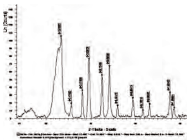
Рис. 2. Дифрактограмма образца Cu(II) / ПААГ
