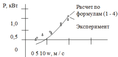
Рис. 1. Вырабатываемая электрическая мощность P в зависимости от скорости ветра w с радиусом горизонтального ветроколеса 1,4 м по расчету по формулам (1 - 4) в сравнении с результатами испытаний ветрогенератора на постоянных магнитах LOW WIND - 1 / 1,5 [5].
