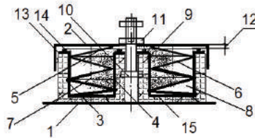
Рис.3. Тарельчатый виброизолятор для технологического оборудования.
