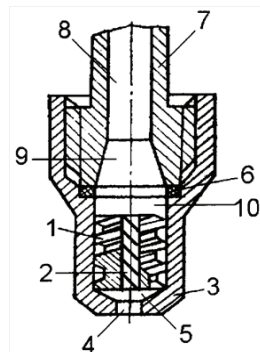
Рис.2. Центробежная форсунка оросительного устройства аппаратов кипящего слоя 3 и 7.
