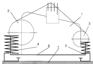
Рис.1. Расчетная схема системы виброизоляции для ткацких станков: 1–станок; 2–навой; 3–товарный валик; 4,5–резиновые виброизоляторы со стороны навоя станка и со стороны грудницы; 6–опорная поверхность станка; 7–межэтажное перекрытие.
