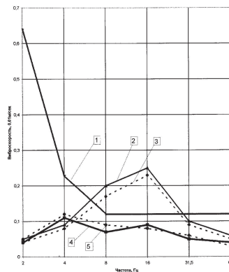
Рис.4. Результаты испытаний системы виброизоляции ткацких станков.
