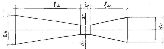
Рис. 1. Расчетная схема трубы Вентури.
