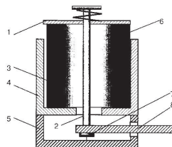
Рис.1. Расчетная схема системы виброизоляции для ткацких станков: 1–станок; 2–навой; 3–товарный валик; 4,5–резиновые виброизоляторы со стороны навоя станка и со стороны грудницы; 6–опорная поверхность станка; 7–межэтажное перекрытие.
