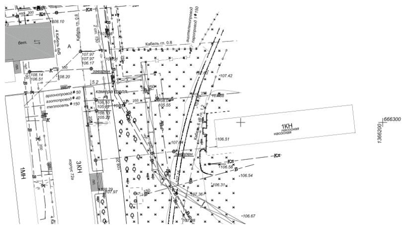
Рисунок 1. Фрагмент топографического плана.
