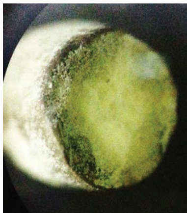
Рис.5. Получение металлической формы палладия на катализаторе методом прогрева его до 250^{\circ}\text{C} в среде водорода
