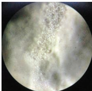
Рис.6. Краевая область палладиевого катализатора, восстановленного в жидкой фазе гипофосфитом натрия (x60)
