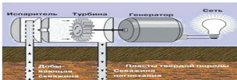
Рисунок 2 - Принцип работы геотермальной электростанции с непрямым типом производства энергии
