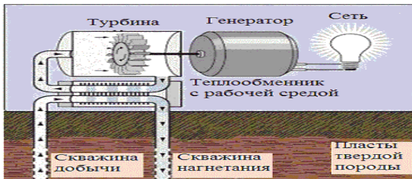
Рисунок 3 - Принцип работы геотермальной электростанции с бинарным циклом
