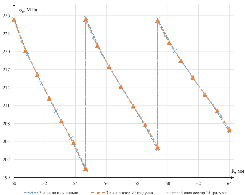
Рис. 8. График распределения кольцевых напряжений для трехслойного цилиндра
