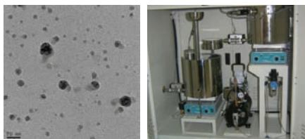
Рис. 1 Типичный ТЕМ снимок наночастиц углерода (слева), получаемый на установке синтеза наночастиц углерода с привитыми карбоксильными группами (справа)
