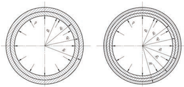
Рис. 1. Исходные схемы нагружения цилиндрических конструкций внутренним давлением а – схема двухслойного цилиндра, б – схема трехслойного цилиндра
