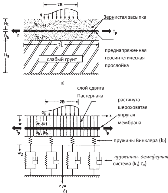
Рис. 2. Модель армированного основания Shukla и Chandra:
