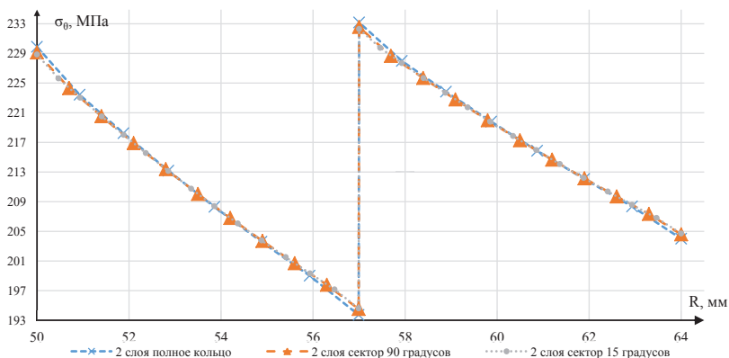
Рис. 7. График распределения кольцевых напряжений для двухслойного цилиндра
