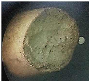
Рис.3. Палладиевый катализатор, обработанный расплавом аммония (x60)
