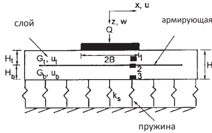
Рис. 1. Модель армированного основания M.R. Madhav и Н.В. Poorooshab
