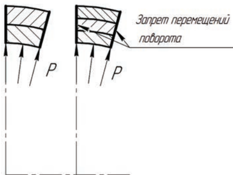
Рис. 5. Расчетная схема для анализа сектора 15^{\circ}
