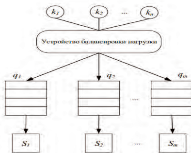
Рис. 1. Схема модели распределенной обработки триггер - запросов в АСУЭО.
