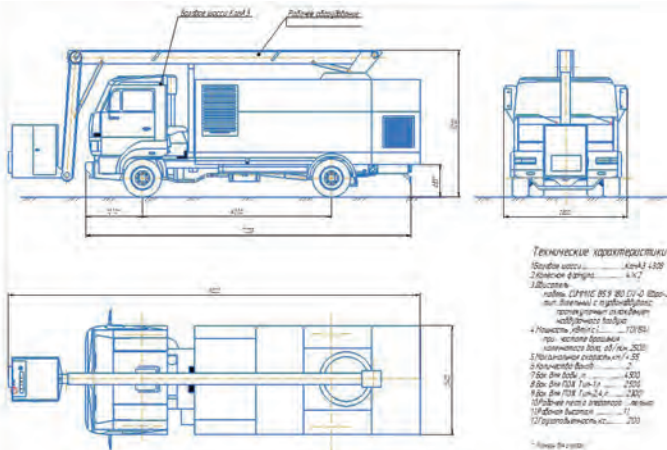
Рисунок 1. Аэродинамическая спецмашина для противоблужденительной обработки ВС
