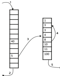
Рис. 2. Графическое изображение работы усовершенствованного алгоритма наименьшей очереди.
