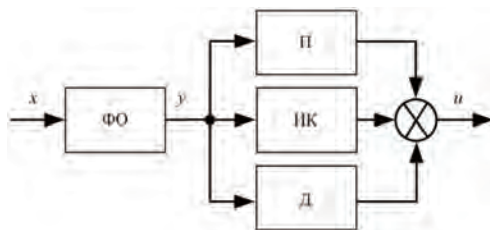
Рис.1. Регулятор
