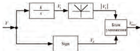
Рис.4. Интегратор Клэгга
